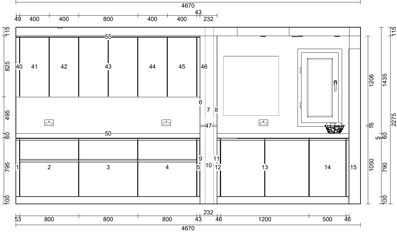
Elevation A/A
